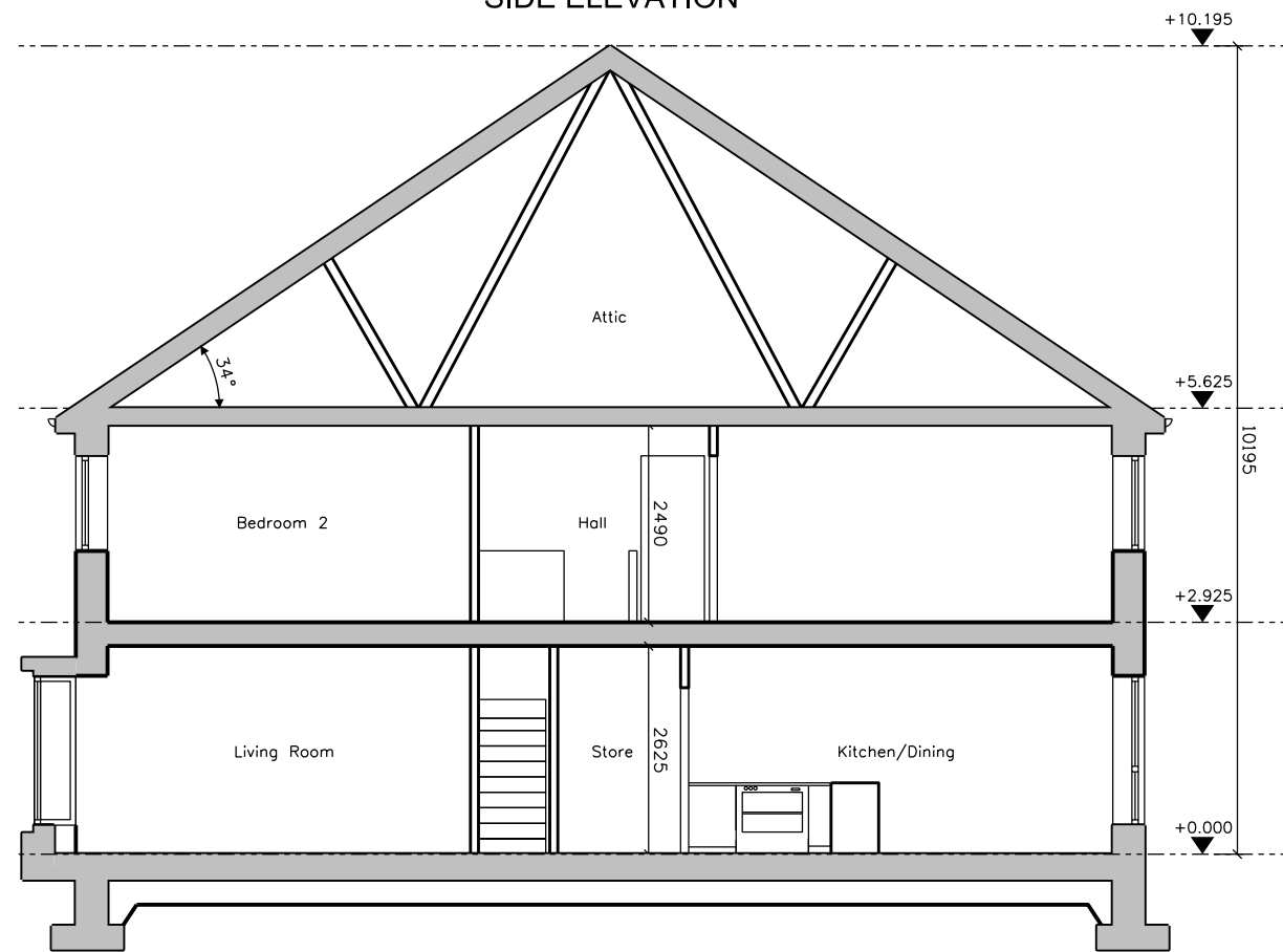
SECTION A-A
